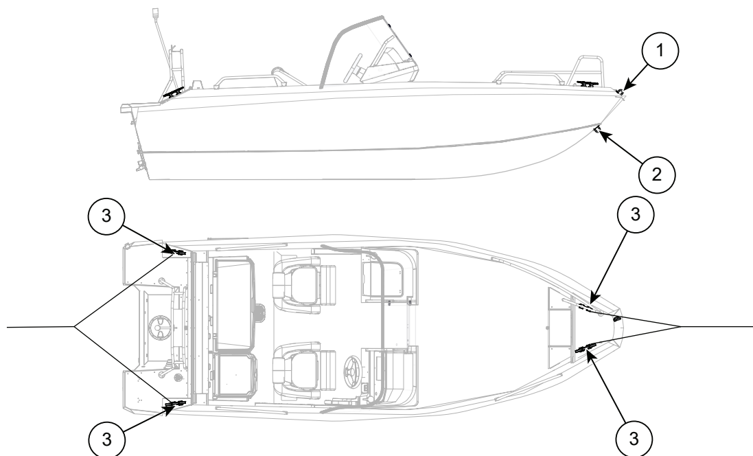
Figur 5.4 Buster LX förtöjnings- och bogseringspunkter
