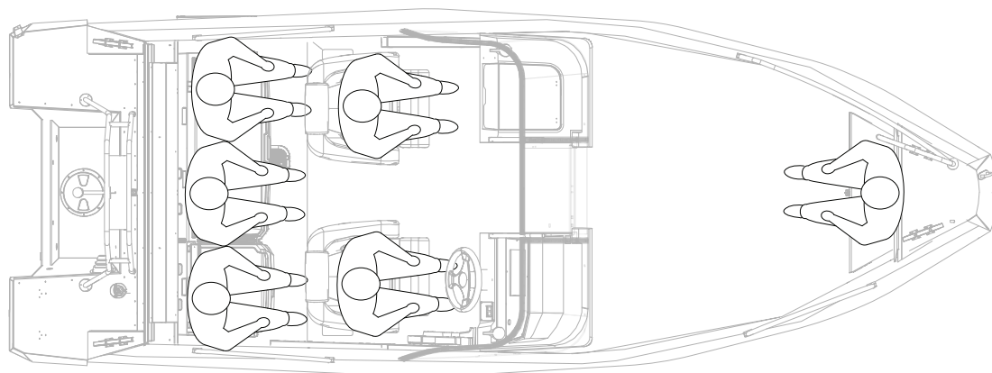
Figur 4.1 Buster LX säten för högst sex (6) passagerare
