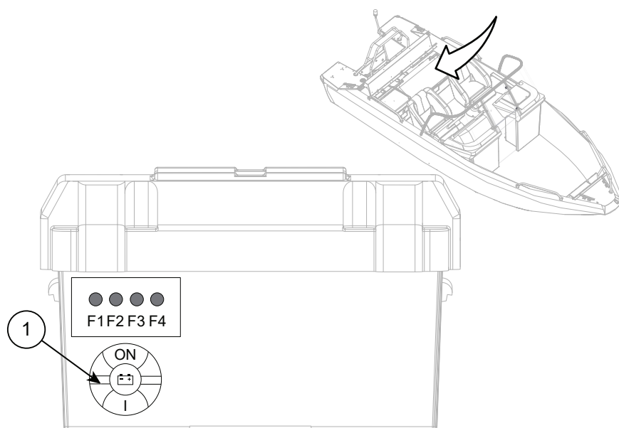
Figur 8.1 Buster LX - huvudströmbrytare och säkringspanel
