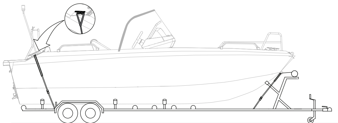
Figur 12.1 Buster LX - släpvagnstransport
