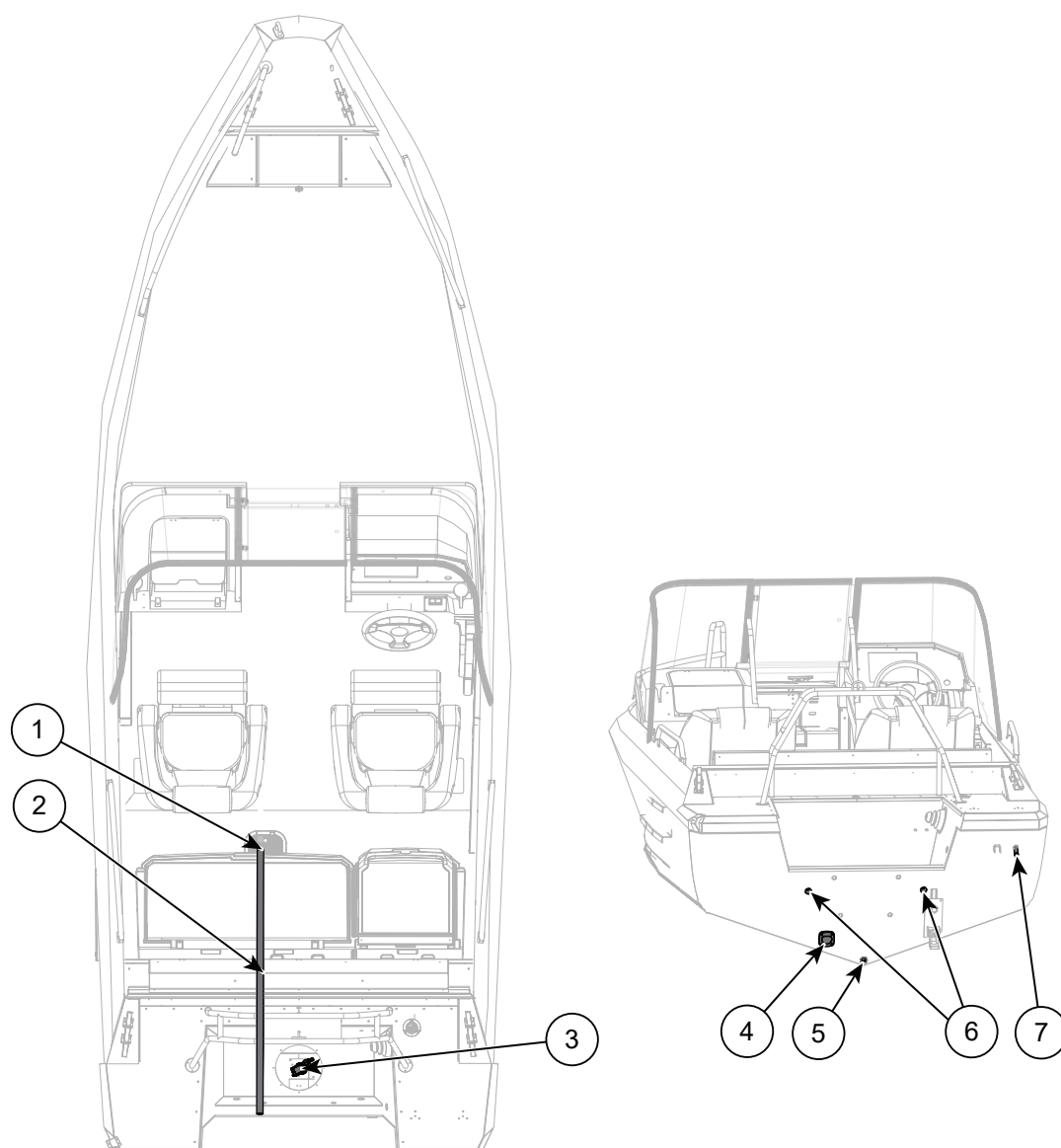
Figur 9.1 Buster LX dräneringsutrustning
